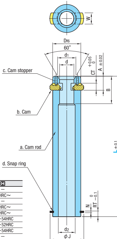
② Cam rod C-ERSR
